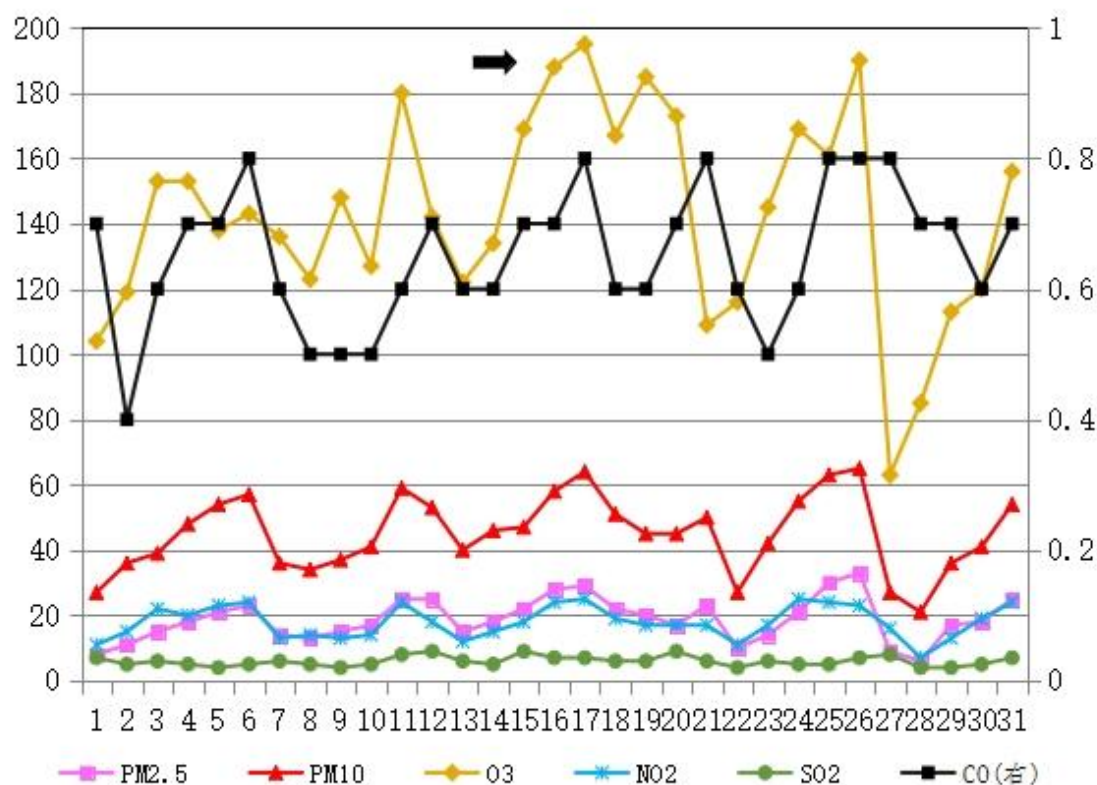
图 1 8 月份鄂州市城区六项污染物日浓度变化趋势
