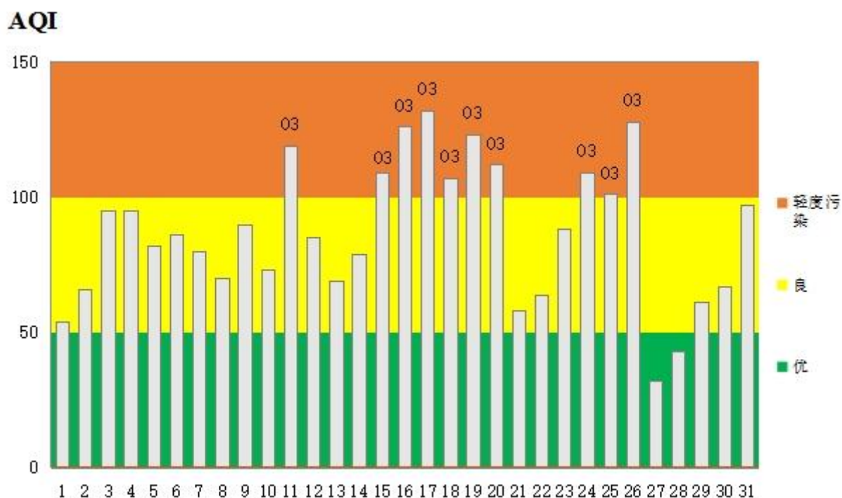
图 2 2023 年 8 月鄂州市区空气质量指数分布图
