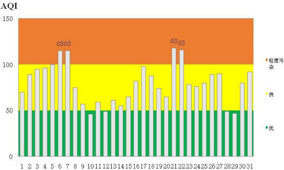
图 2 2022 年 5 月鄂州市区空气质量指数分布图
