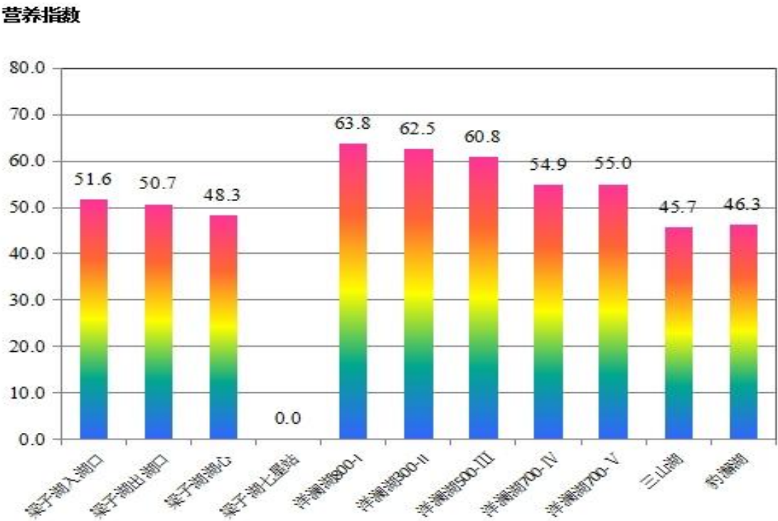
图 4 梁子湖、三山湖、豹澥湖、洋澜湖营养指数图
