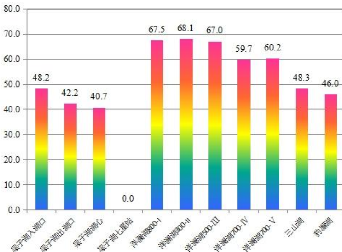
图 4 梁子湖、三山湖、豹澥湖、洋澜湖营养指数图
