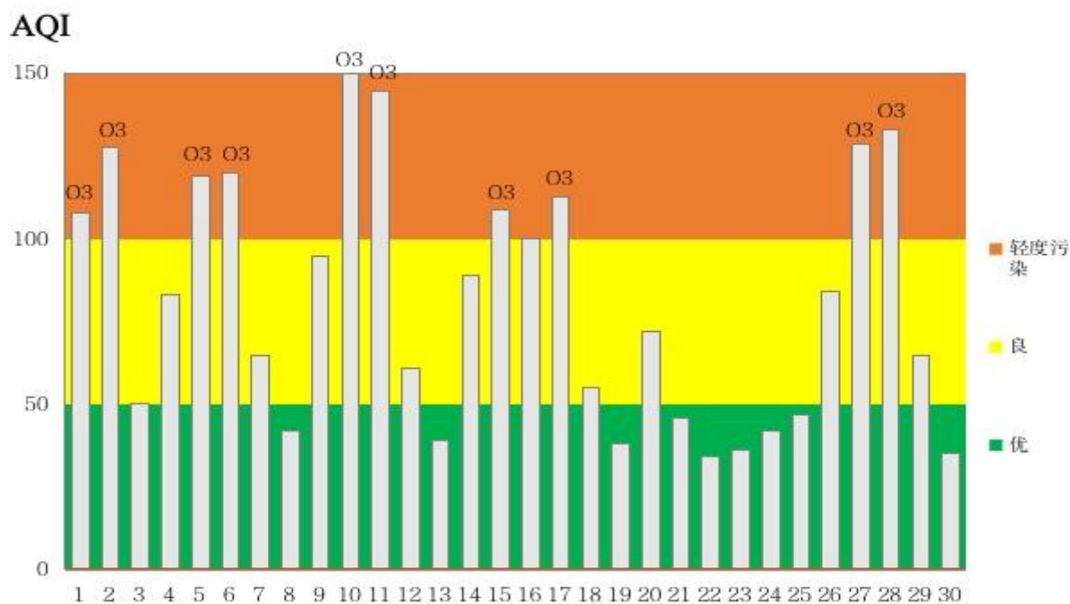
图 2 2026 年 6 月鄂州市区空气质量指数分布图
