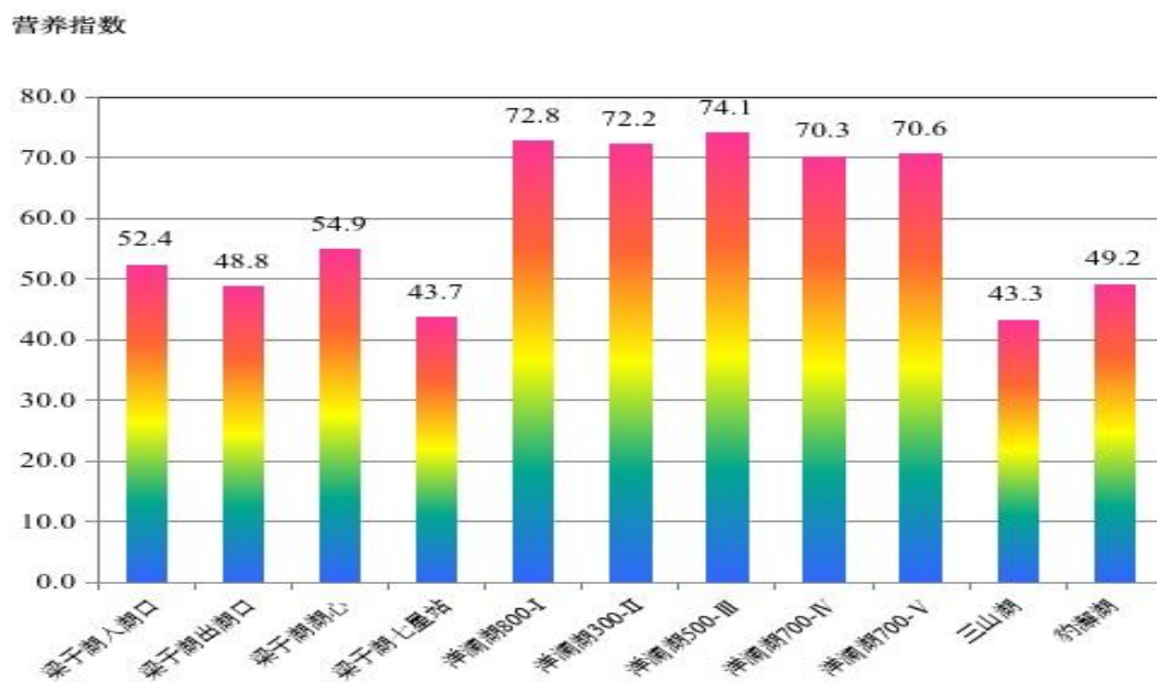
图 4 梁子湖、三山湖、豹澥湖、洋澜湖营养指数图
