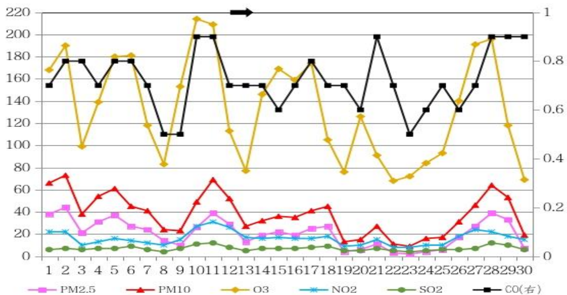
图 1 6 月份鄂州市城区六项污染物日浓度变化趋势
