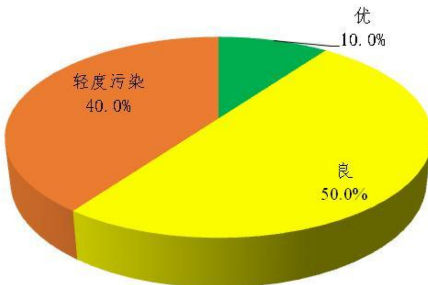
图2 2021年9月鄂州市区空气质量指数分布图
