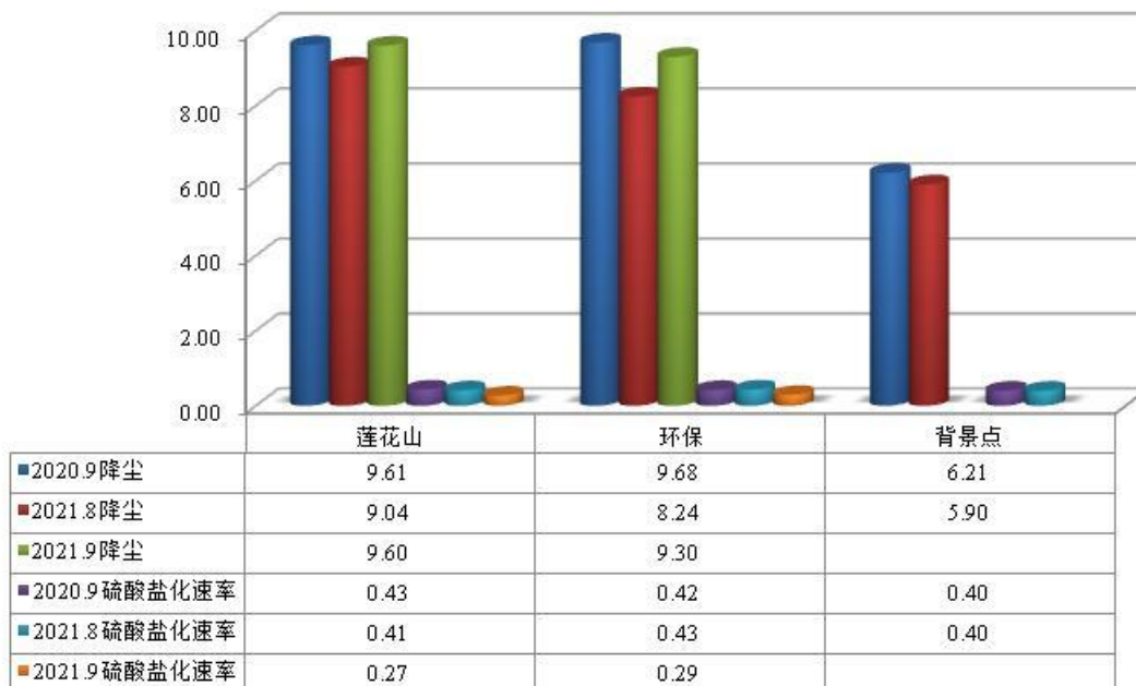
图 5：城区 9 月降尘及硫酸盐化速率
