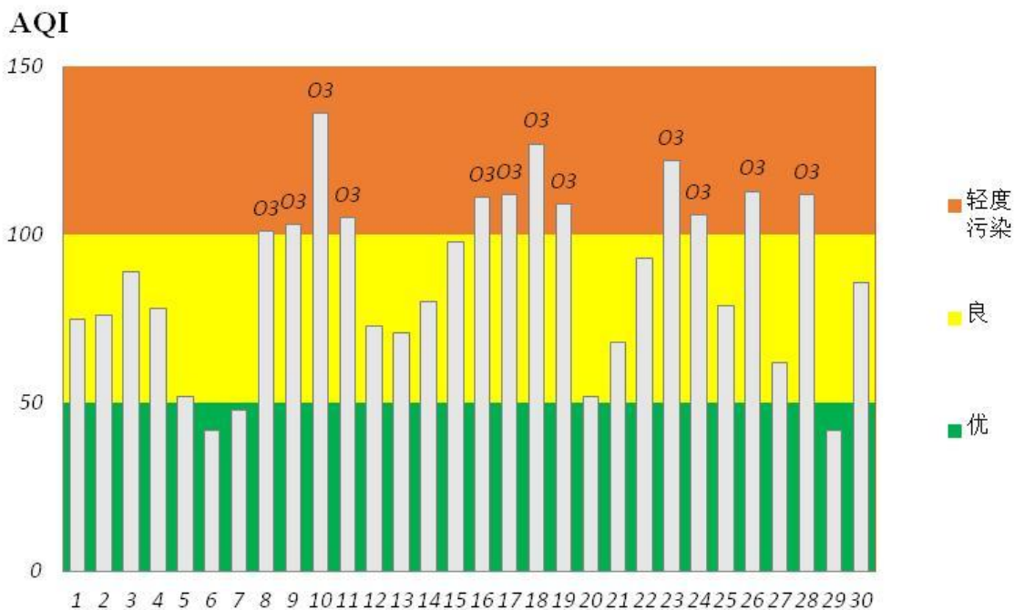
图2 2021年9月鄂州市区空气质量指数分布图
