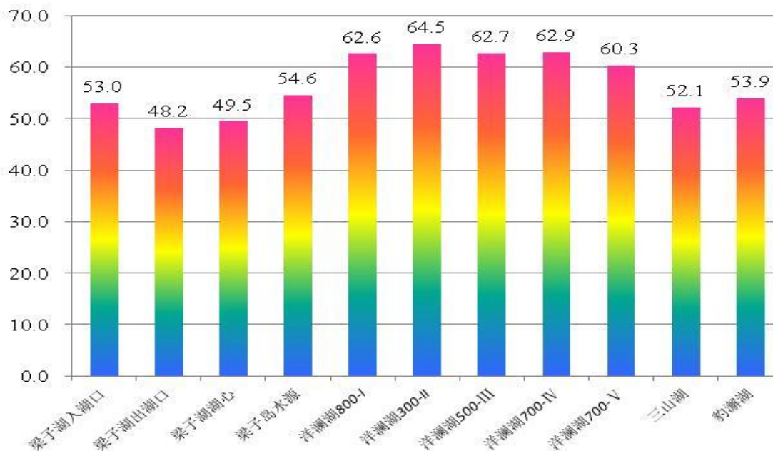
营养指数 图4 梁子湖、洋澜湖、三山湖、豹澥湖营养指数图
