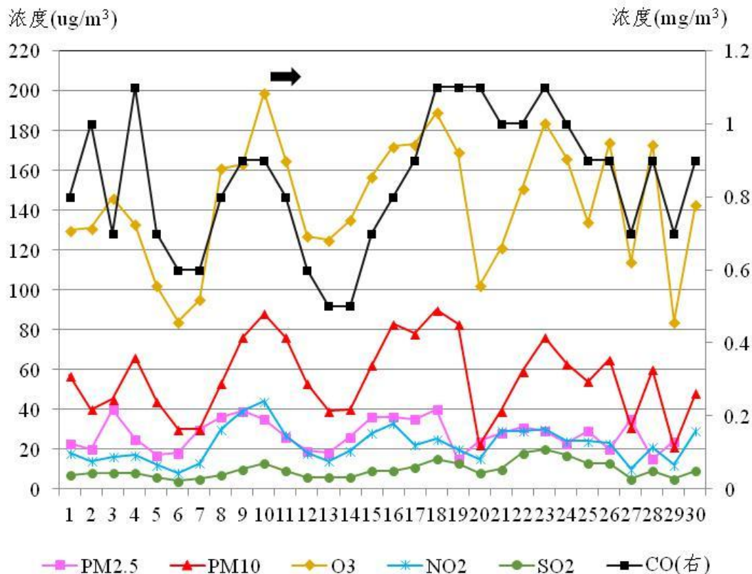
图1 9月份鄂州市城区六项污染物日浓度变化趋势
