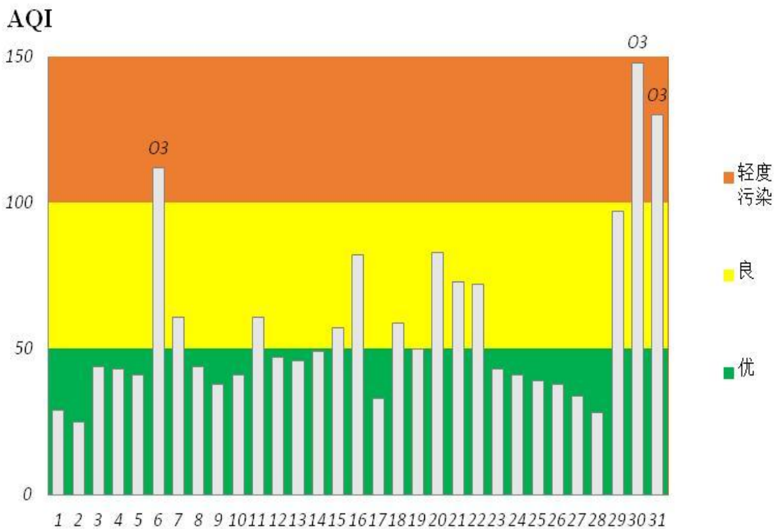
图2 2021年7月鄂州市区空气质量指数分布图
