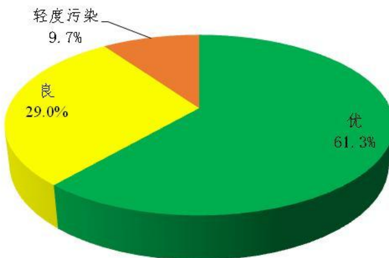
图2 2021年7月鄂州市区空气质量指数分布图
