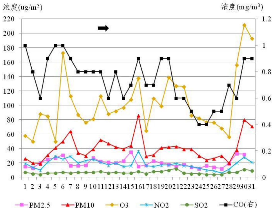
图1 7月份鄂州市城区六项污染物日浓度变化趋势
