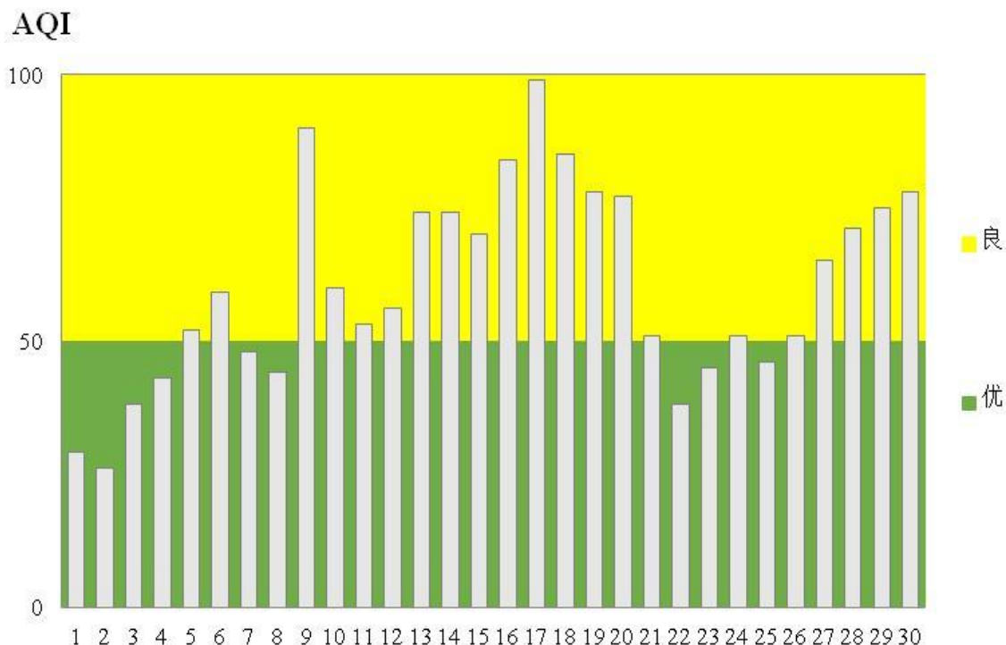
图 2 2021 年 4 月鄂州市区空气质量指数分布图
