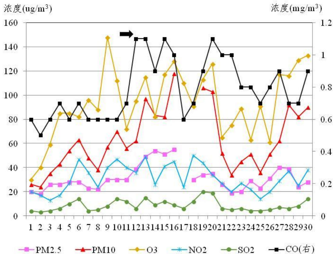
图 1 4 月份鄂州市城区六项污染物日浓度变化趋势
