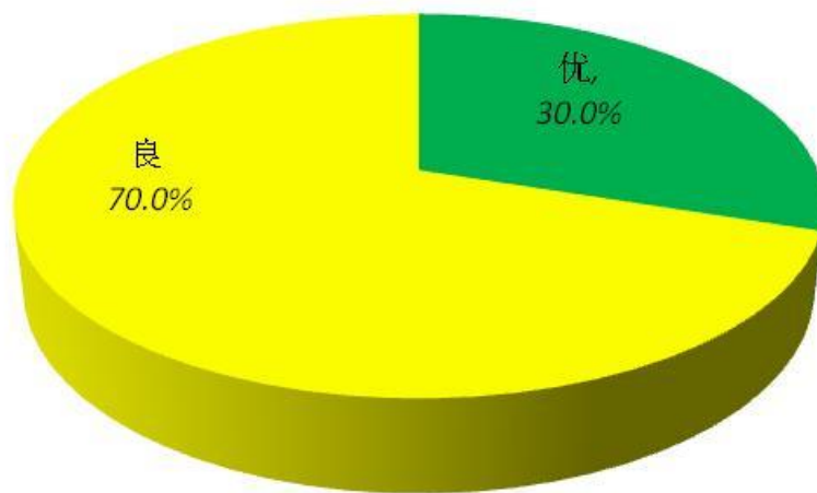
图 3 2021 年 4 月鄂州市区空气质量比例图
