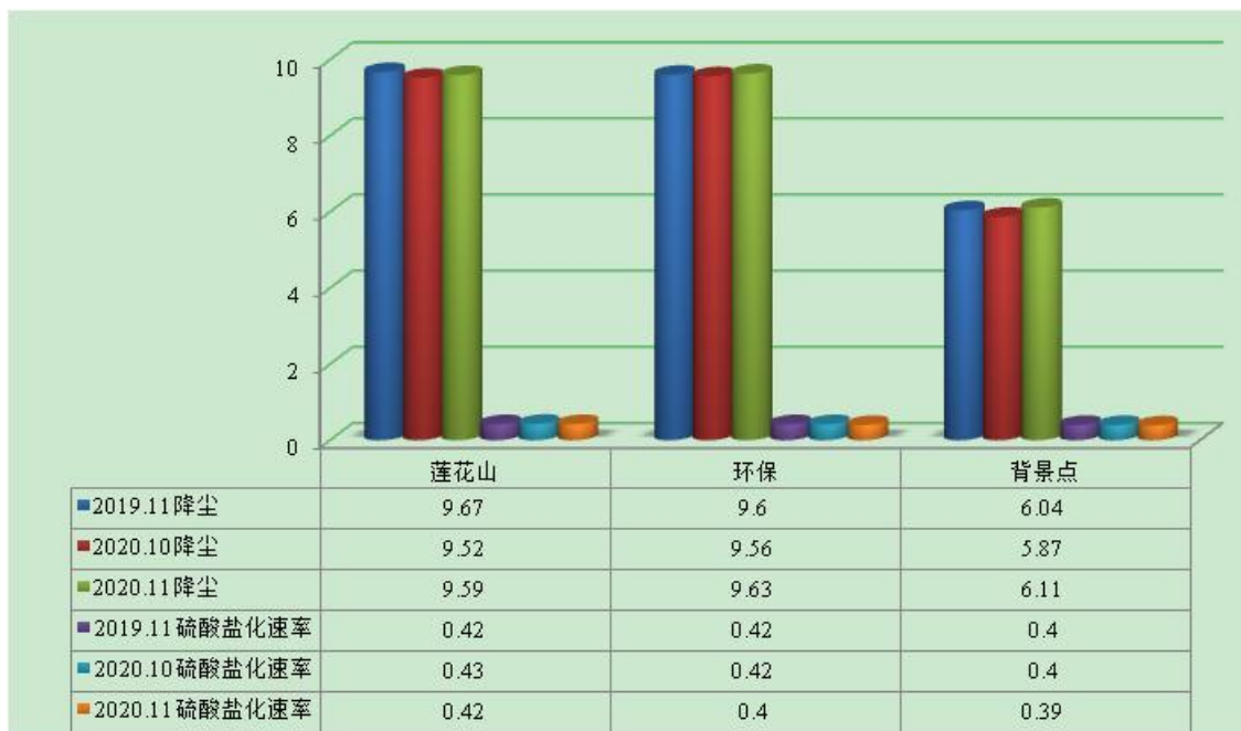
图 5：城区 11 月降尘及硫酸盐化速率
