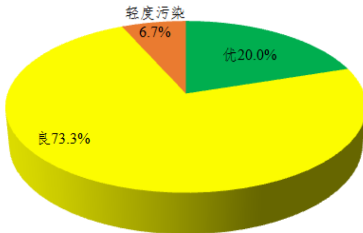
图 2 2020 年 11 月鄂州市区空气质量指数及超标天首要污染物分布图
